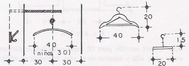
9.2. Tipos de ganchos para ropa y sus medidas.
