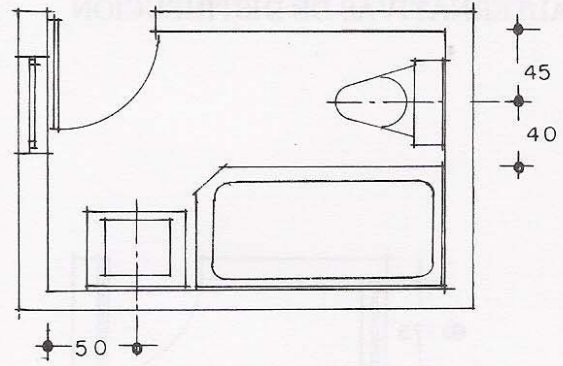
6.18. Baño con tina chica ventilación de lado.
