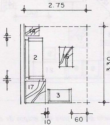
2.11. Disposición en escuadra con mesa al centro como foco de interés en una superficie de 9.07 m 2 .
