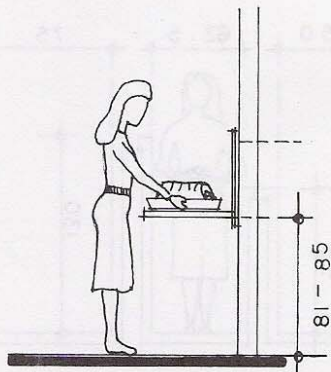
4.3. Altura promedio para la ubicación de hornos empotrados en la pared.
