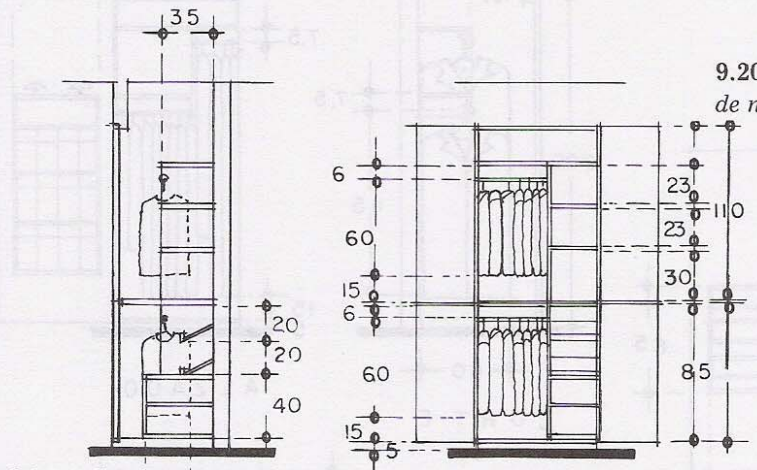
ALZADO
