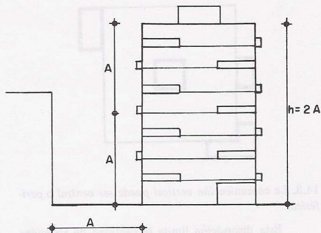
14.1. La relación de altura del edificio va en función de la distancia al paramento del edificio más próximo.
