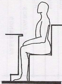
1.16.(B) Distancia mínima entre el coxis y la rodilla (asientos o bancas fijas al piso).
