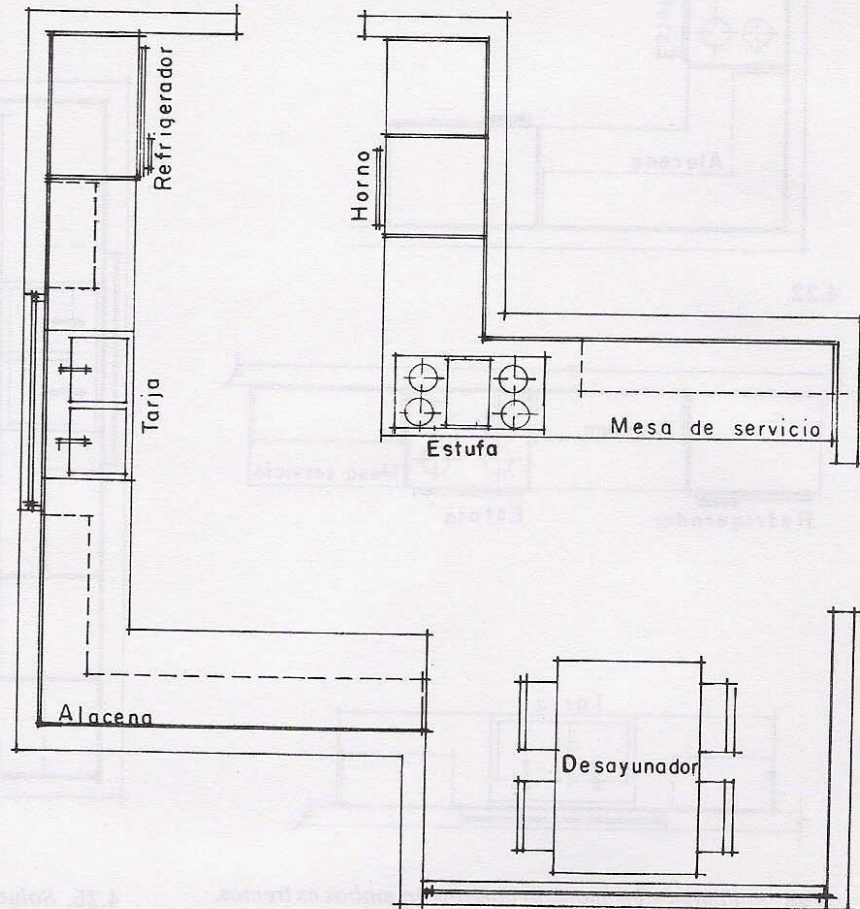
4.27. Solución en "S" con desayunador.
