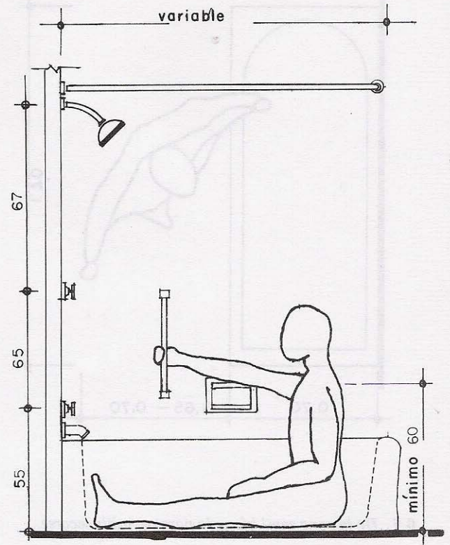
6.5. Medidas recomendables en el uso de la tina.
