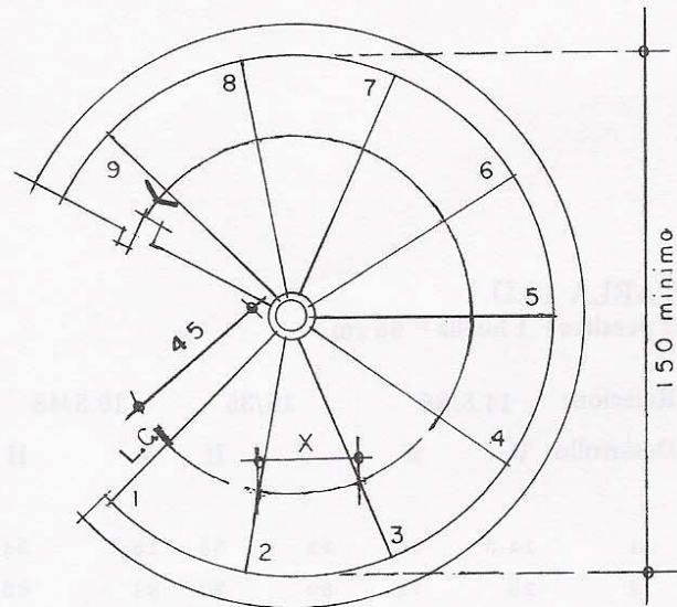
COMPENSACION DE UNA ESCALERA
