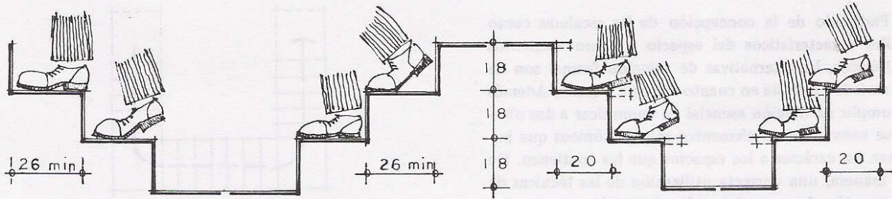
SOLUCION POSIBLE SIN NARIZ
