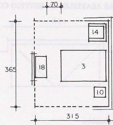
5.19. Cama matrimonial con sillón individual. 11.49 m 2
