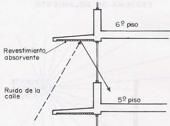
13.25. El ruido reflejado en los elementos de protección solar puede ser evitado con un revestimiento absorbente.
