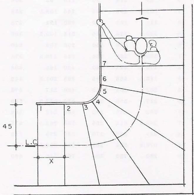
COMPENSACION DE UNA ESCALERA
