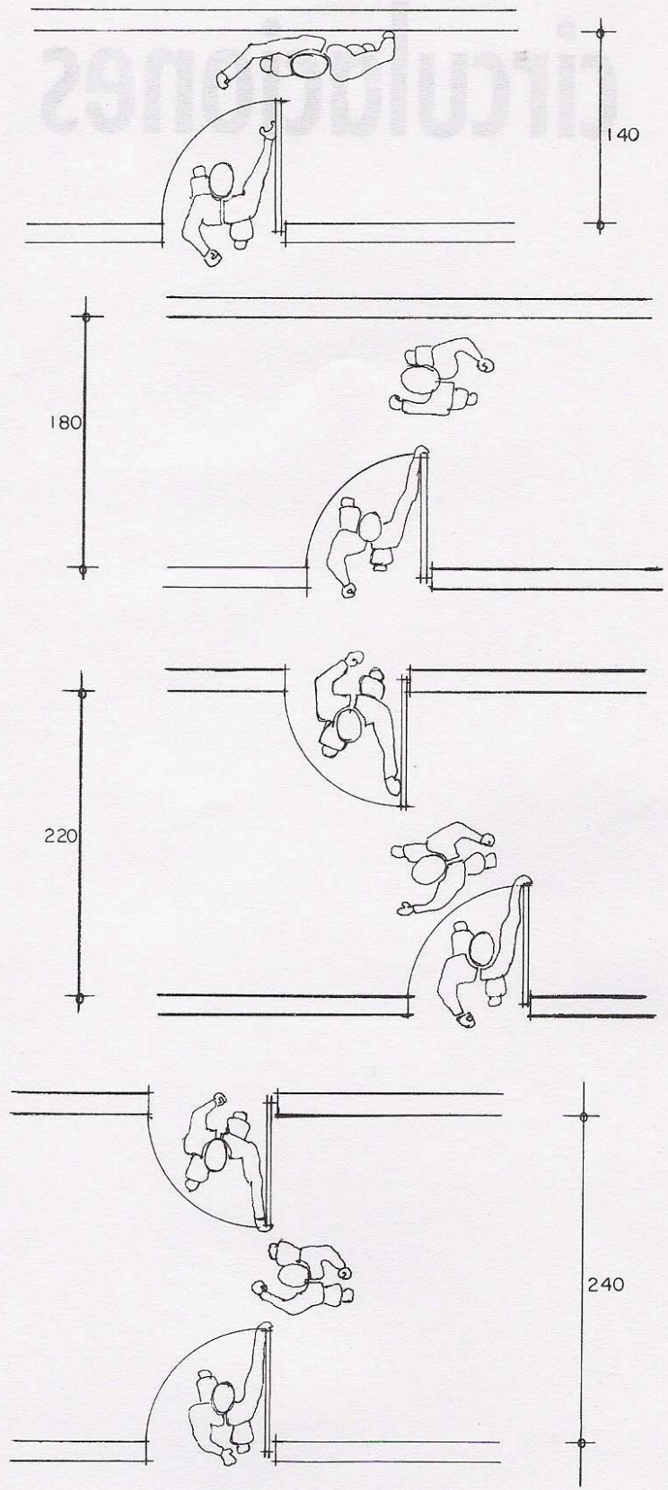
13.2. Espacios para circulación con obstrucciones.
