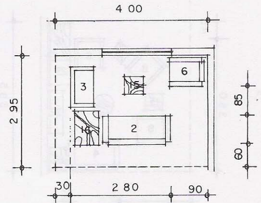
2.15. Grupo primario de conversación; la ventana es un foco de interés. El área es de 11.80 m 2 .
