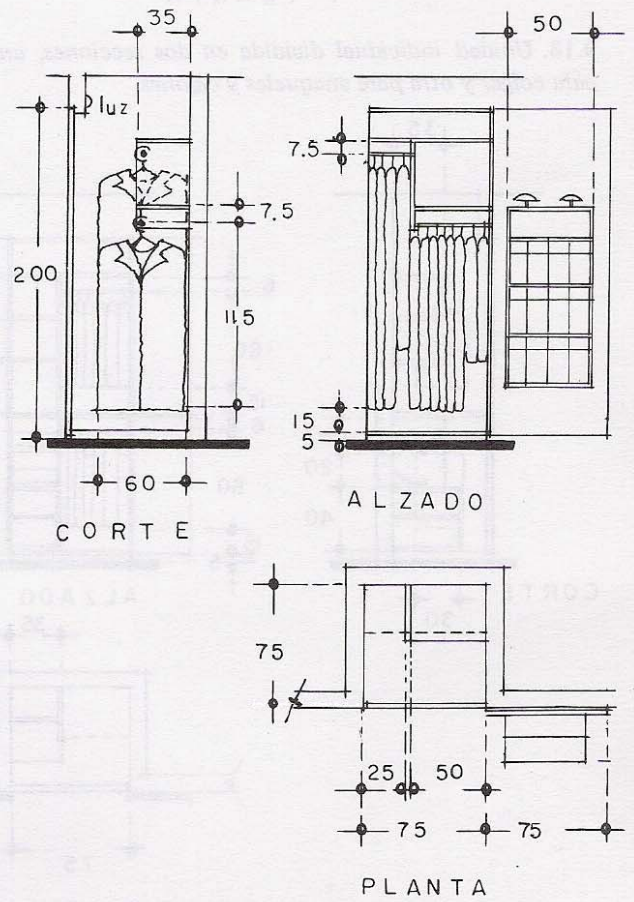
9.17. Closet individual con dos tubos para colgar a diferente nivel. La puerta se usa para sombreros y zapatos.
