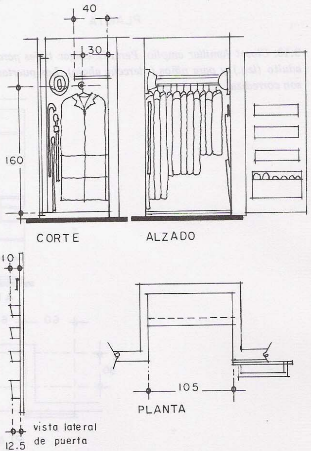
9.12. Closet masculino sin anaqueles. Las cajas de la parte interior de la puerta se usan para calcetines y zapatos.
