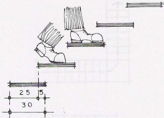
SOLUCION POSIBLE SIN NARIZ
