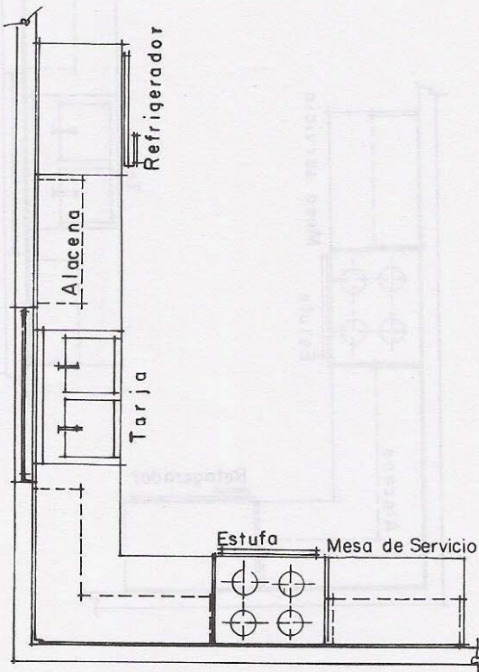
4.17. Soluciones sencillas en forma de "L".
