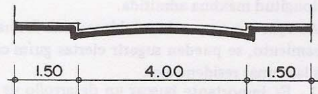
15.3. Diferentes anchos y alternativas de calles.
