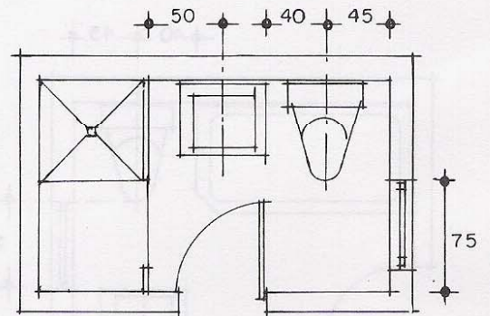
6.14. Baño chico con regadera y zona vestidor.
