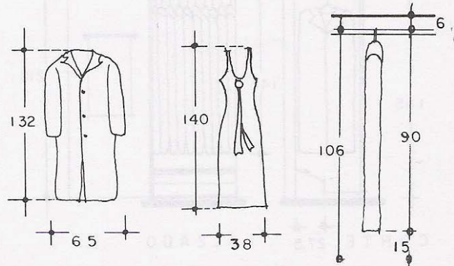
9.1. Medidas de los objetos más comunes que se pueden guardar en los closets.
