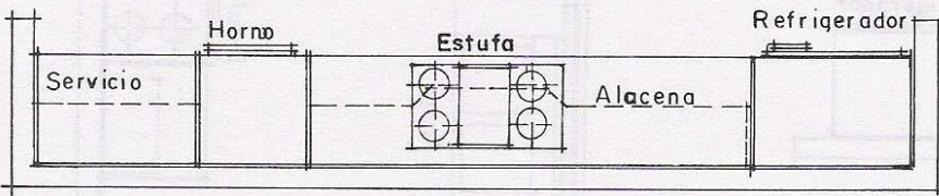
4.26. Disposición en paralelo de una planta rectangular. El ancho se reduce al mínimo. Permite incluir desayunador para 2 ó 3 personas.
