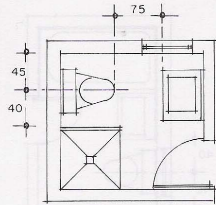
6.12. Baño chico con regadera en esquina.
