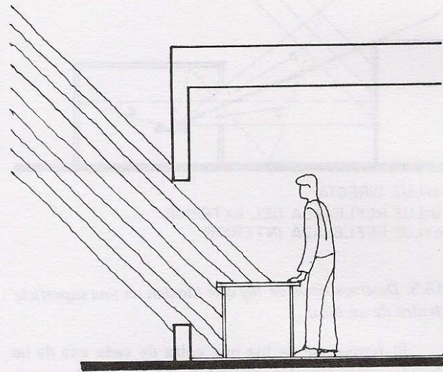
13.9. El efecto de la luz en ventanas con distinta altura.
