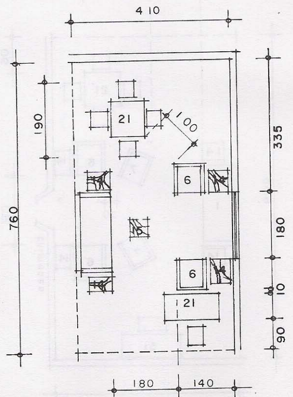
2.26. Un grupo grande cortado por una circulación central que comunica al escritorio (21) y a la mesa de juego. 31 m 2 .
