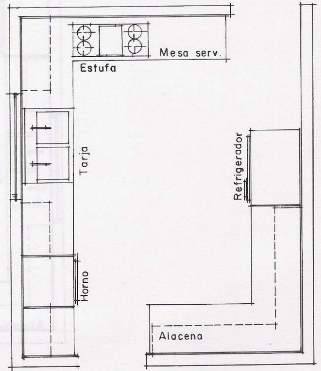
4.25. Solución en doble "L".
