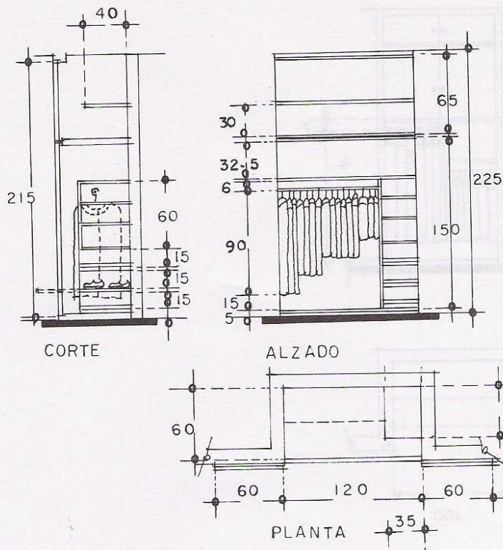
9.10. Closet, para niños, con cajones, anaqueles y espacio para colgar trajes.
