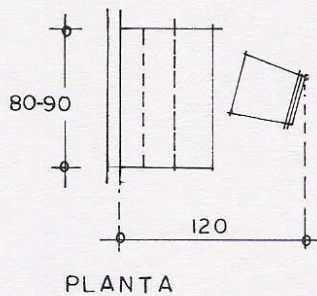
7.4. Espacio mínimo para la utilización de un escritorio y su silla.
