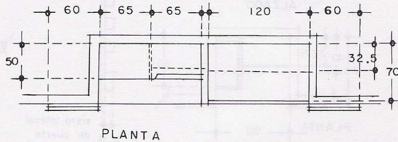
9.14. Closet matrimonial separado en dos secciones, una para cajones y anaqueles y otra para colgar ropa.
