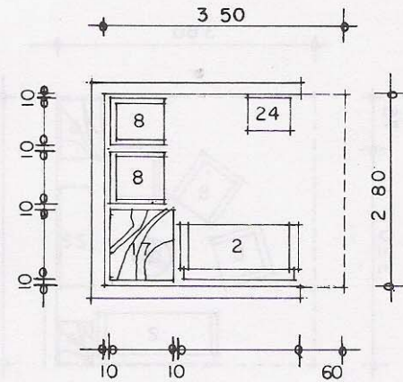
2.14. Solución en escuadra con T.V. y mesa esquinera; superficie de 9.80 m 2 .
