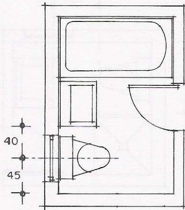
6.15. Baño chico con tina chica, ventilación sobre W.C.
