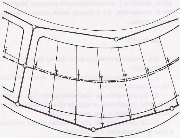
15.6. Afectación de lotes en calles paralelas al contorno.
