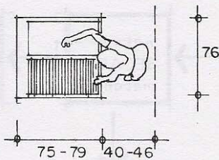
12.3. Espacio necesario para lavar en un lavadero empotrado.
