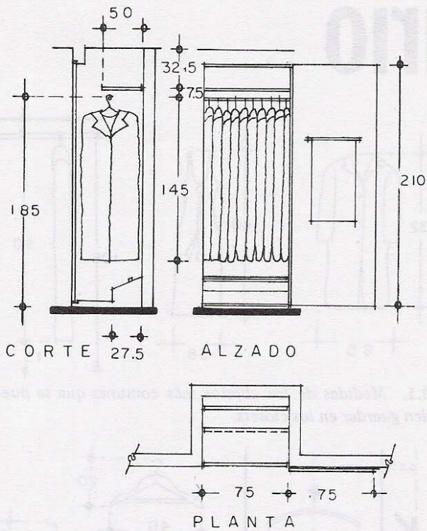
9.5. Closet sencillo para 10 trajes colgados, sombreros en la parte alta y zapatos en el piso; la puerta se utiliza para colgar corbatas y cinturones.
