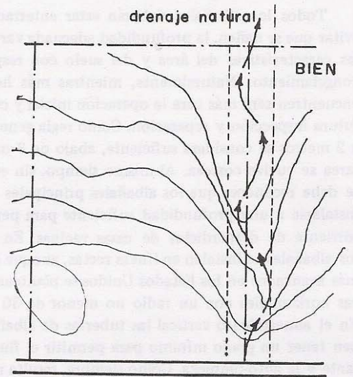
15.7. La ubicación de lotes en curvas de nivel paralelas a la calle aprovechando el drenaje natural del terreno.
