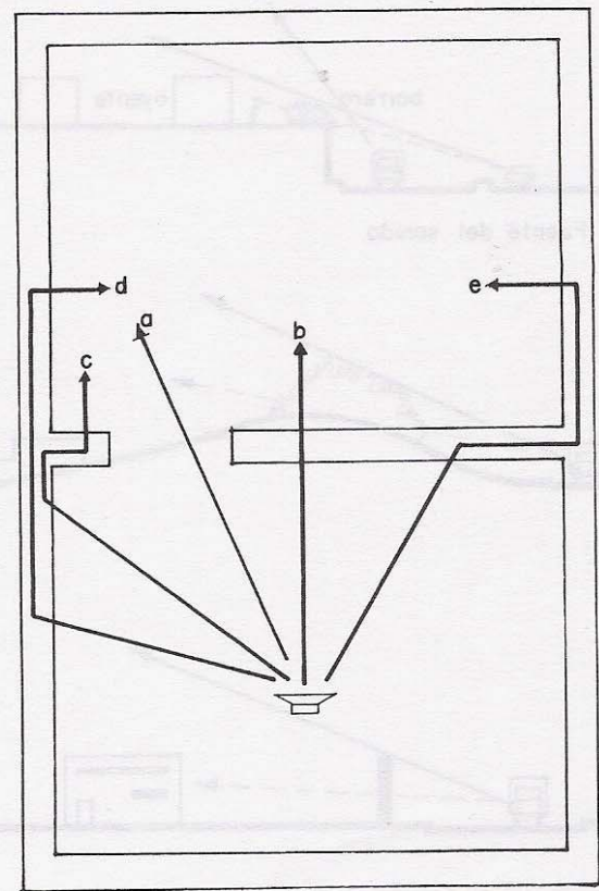
13.21. Transmisión dentro de una estructura del sonido. a) sonido directo, b) a través de un muro, c, d, e, a través de la estructura.
