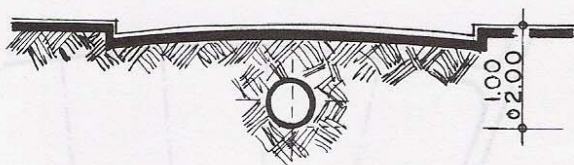
15.9. Profundidad de albañales en calles.
